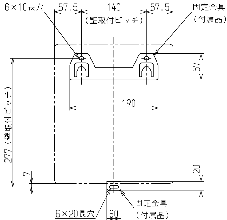
■固定金具詳細図
