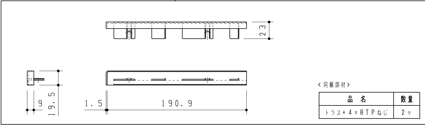
天板キャップセットL ( 奥行小 )
