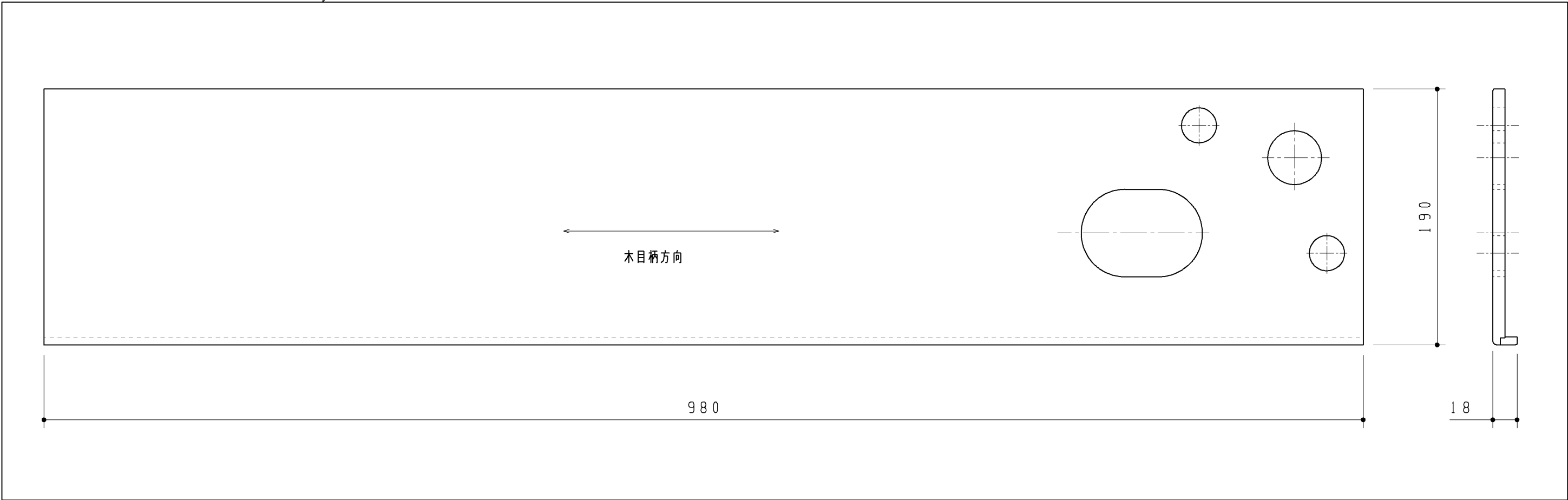
天板キャップセットL ( 奥行小 )
