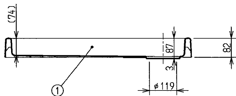
断面A-A
