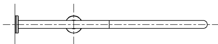
取付座詳細(1:2)
