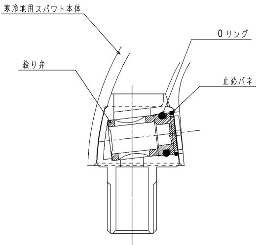
E-E断面詳細図(S=1:1)
