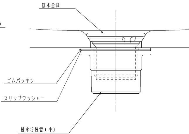
B部詳細図(S=1:1)
