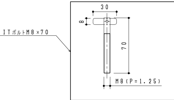
D部詳細図(S=1:1)
