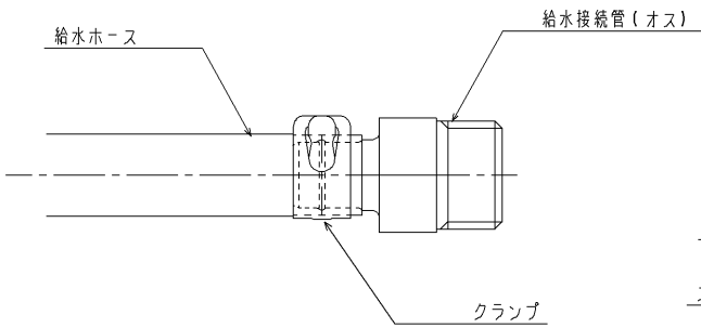
C部詳細図(S=1:1)
