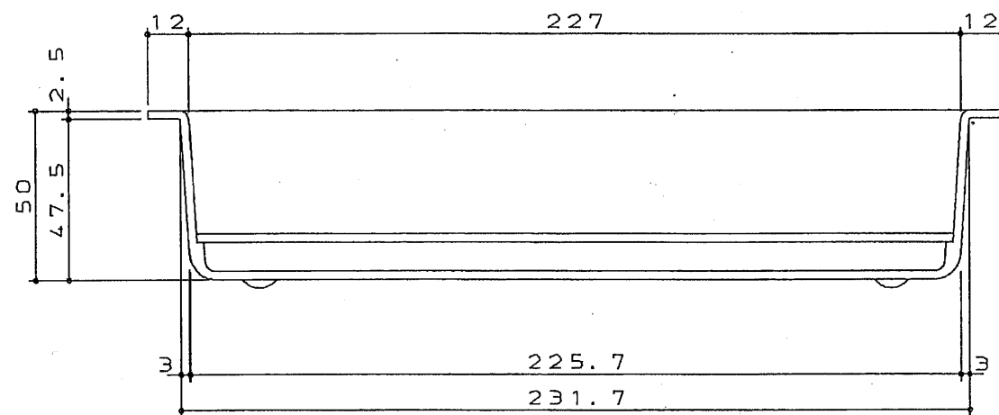
A - A
