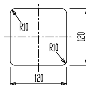
カウンター切込寸法
