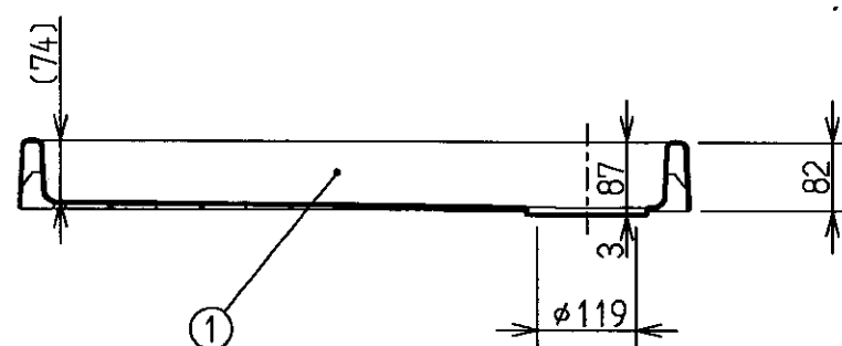
断面A-A
