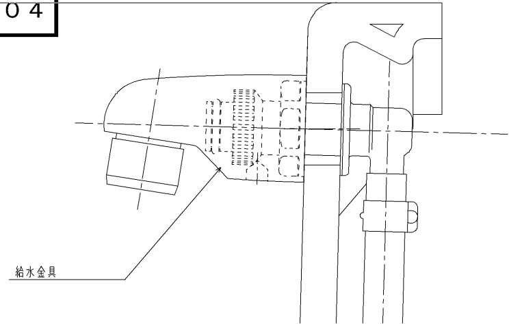
C部詳細図 (S=1:1)
