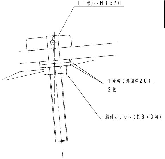
E部詳細図 (S=1:1)
