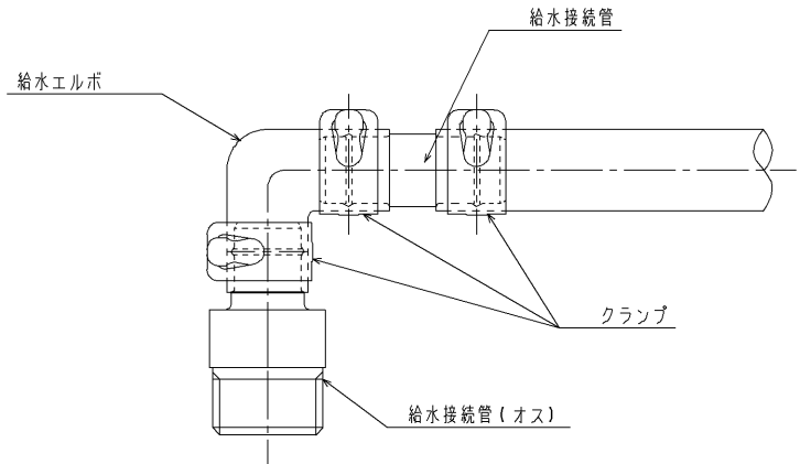
F部詳細図 (S=1:1)
