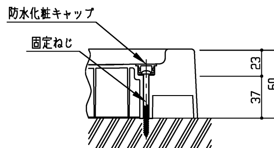
固定部詳細(尺度フリー)
