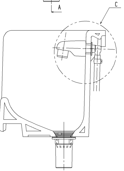
B - B 断面詳細図
