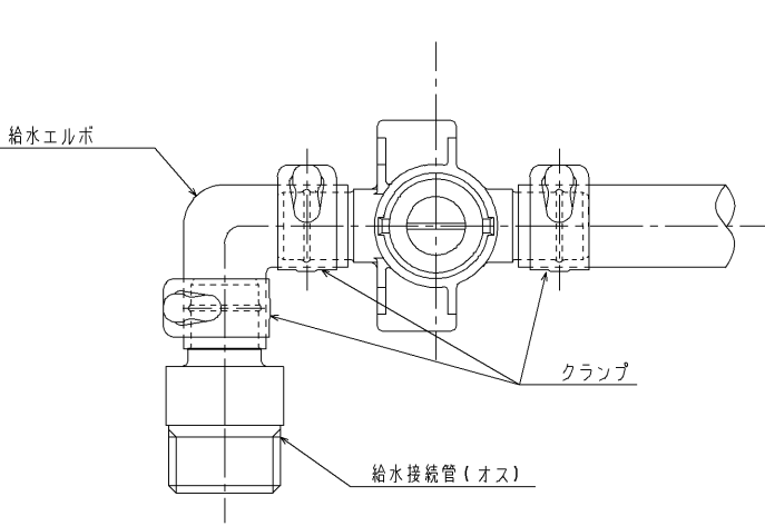
F 部詳細図 (S=1:1)
