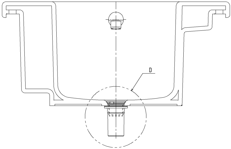
A - A 断面詳細図
