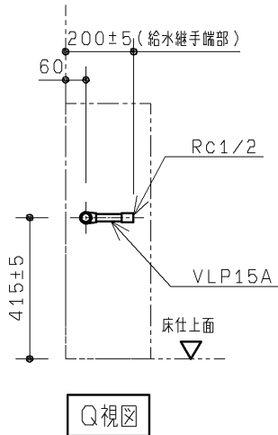
P 視図
