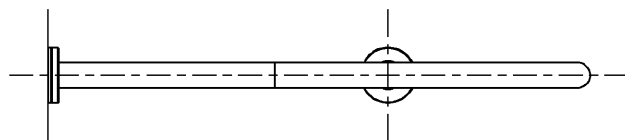
取付座詳細(1:2)
