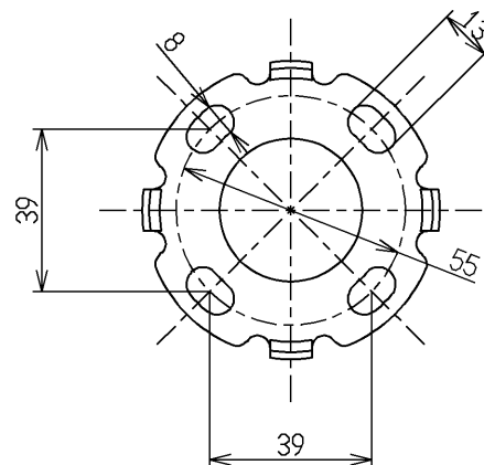
取付座詳細(1:2)
