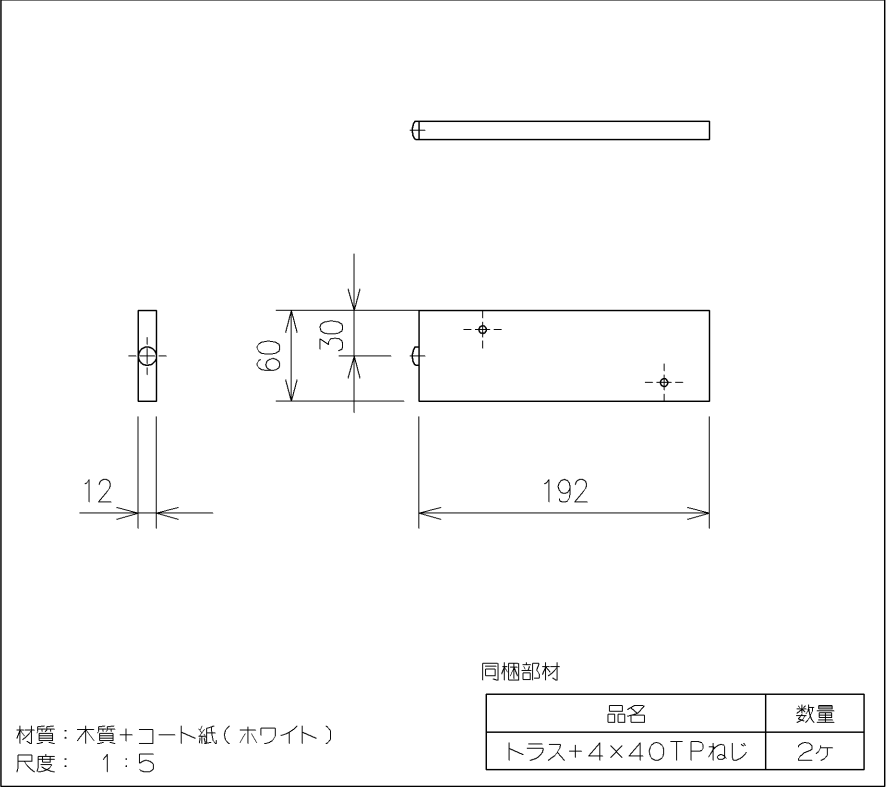
側板組品
