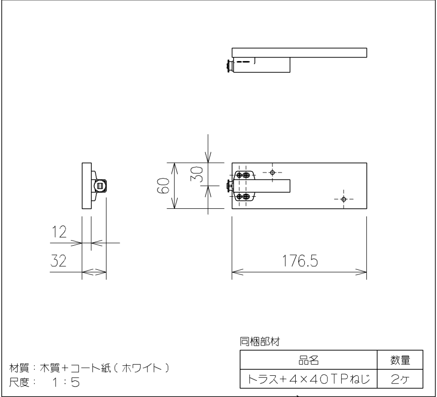
側板組品
