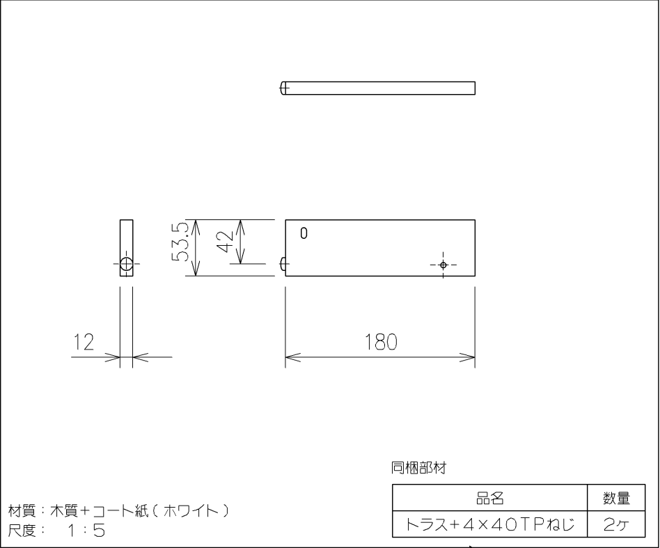
側板組品
