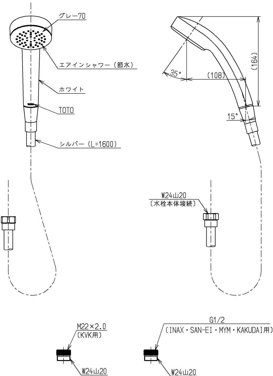
取替え接続用アダプタ
