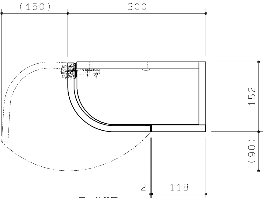
開口状態図
