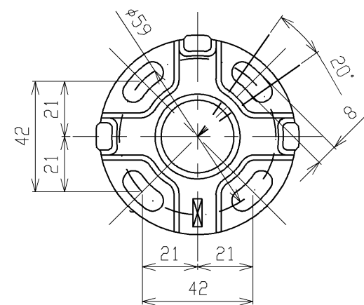
取付座詳細(1:2)
