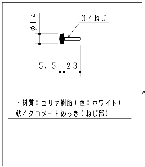
化粧ねじ
