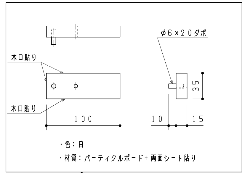
棚板受け材
