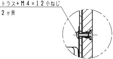
A部詳細 (S=1:2)
