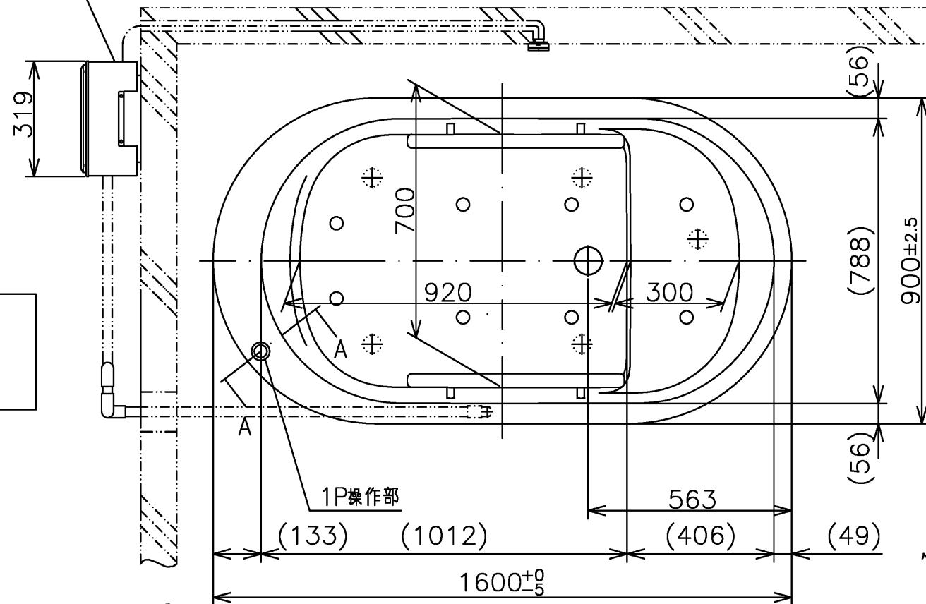
エアブローⅡ機能部
