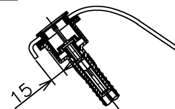
断面A-A(1:5)
