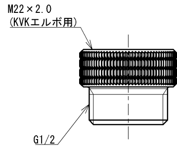
取替え接続用アダプタ
