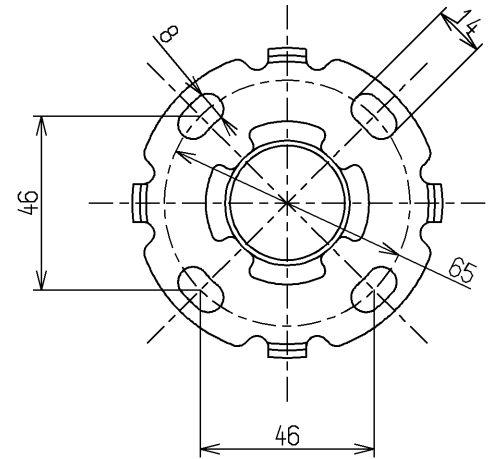
取付座詳細(1:2)
