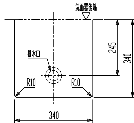
カウンター切込寸法
