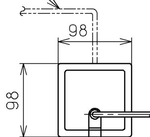
電源ボックス正面視
