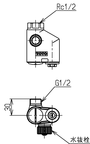
止水栓部(2ヶ)
