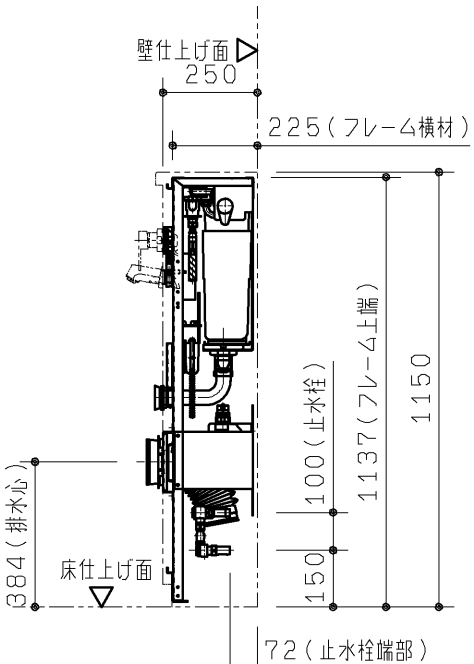
R 視図
