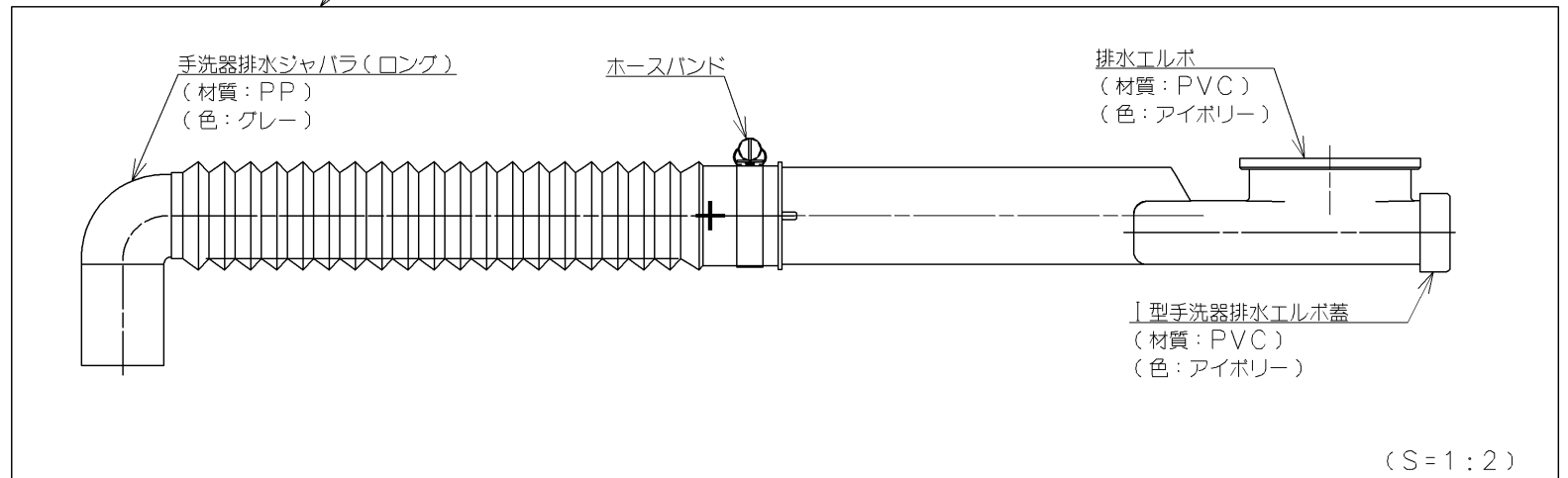
接続管組品
