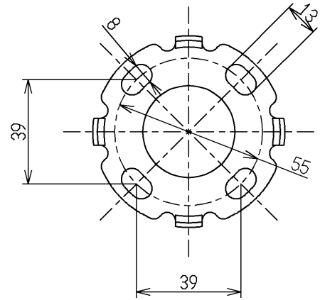
取付座詳細(1:2)
