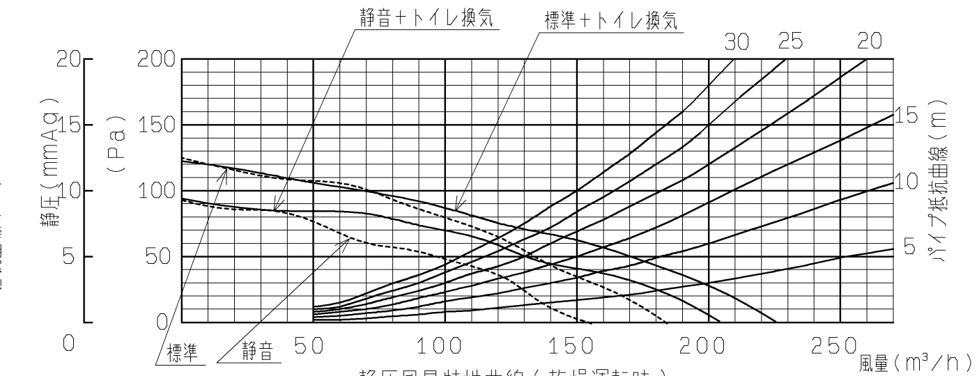
静圧風量特性曲線（乾燥運転時）
