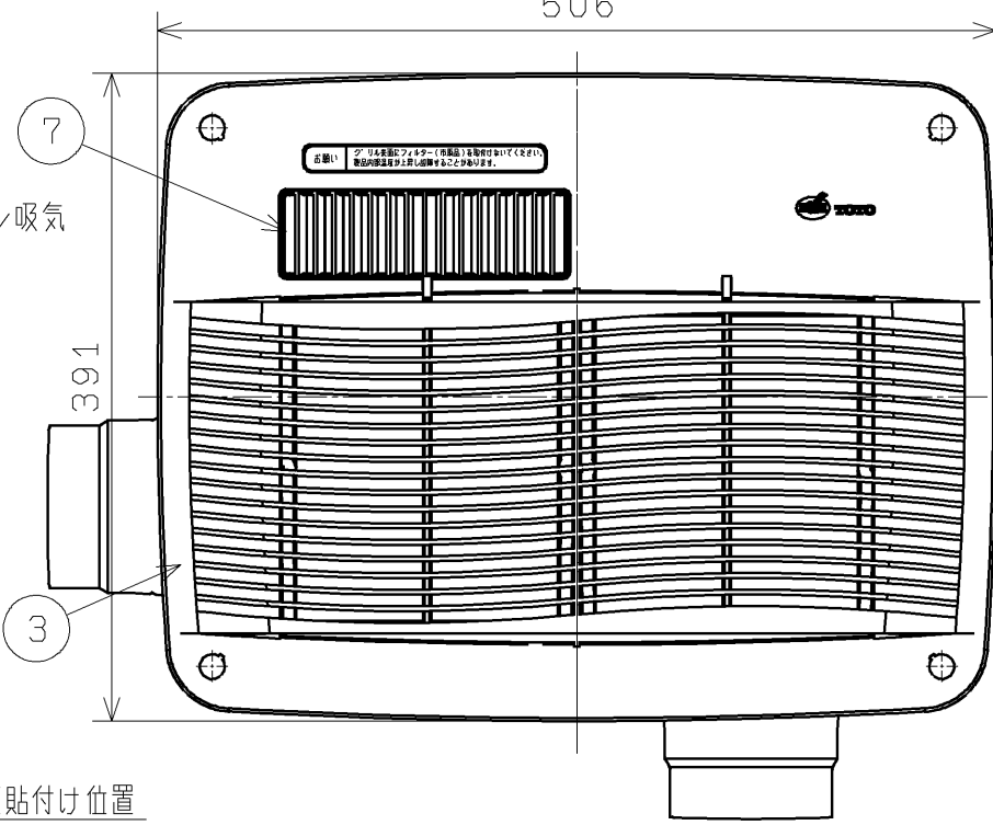
天井取付図 (1:5)
