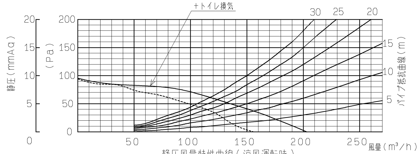
静圧風量特性曲線（涼風運転時）
