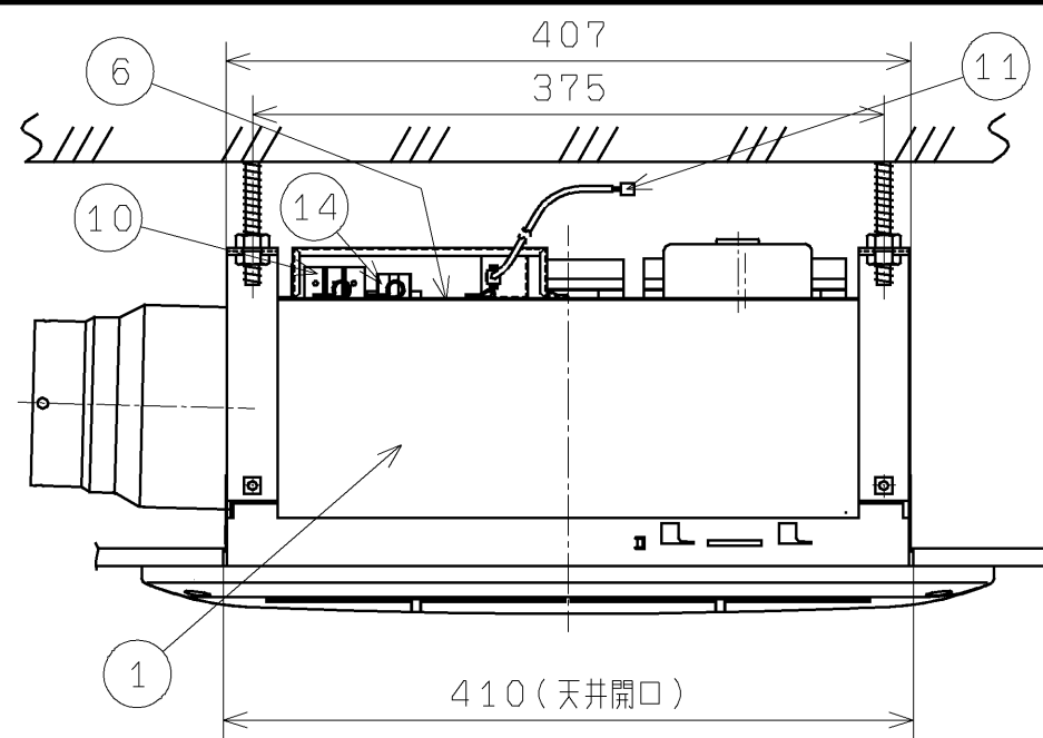
天井取付図 (1:5)
