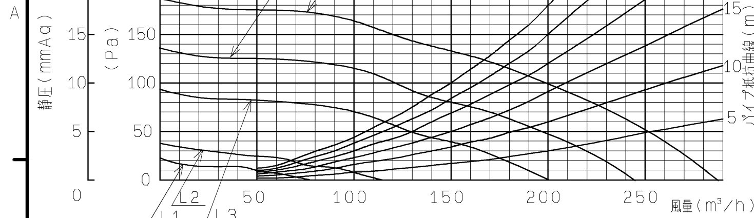
静圧風量特性曲線（24時間換気運転時） ※暖房（入浴前、入浴中）運転時は24時間換気と同じ風量で換気します。
