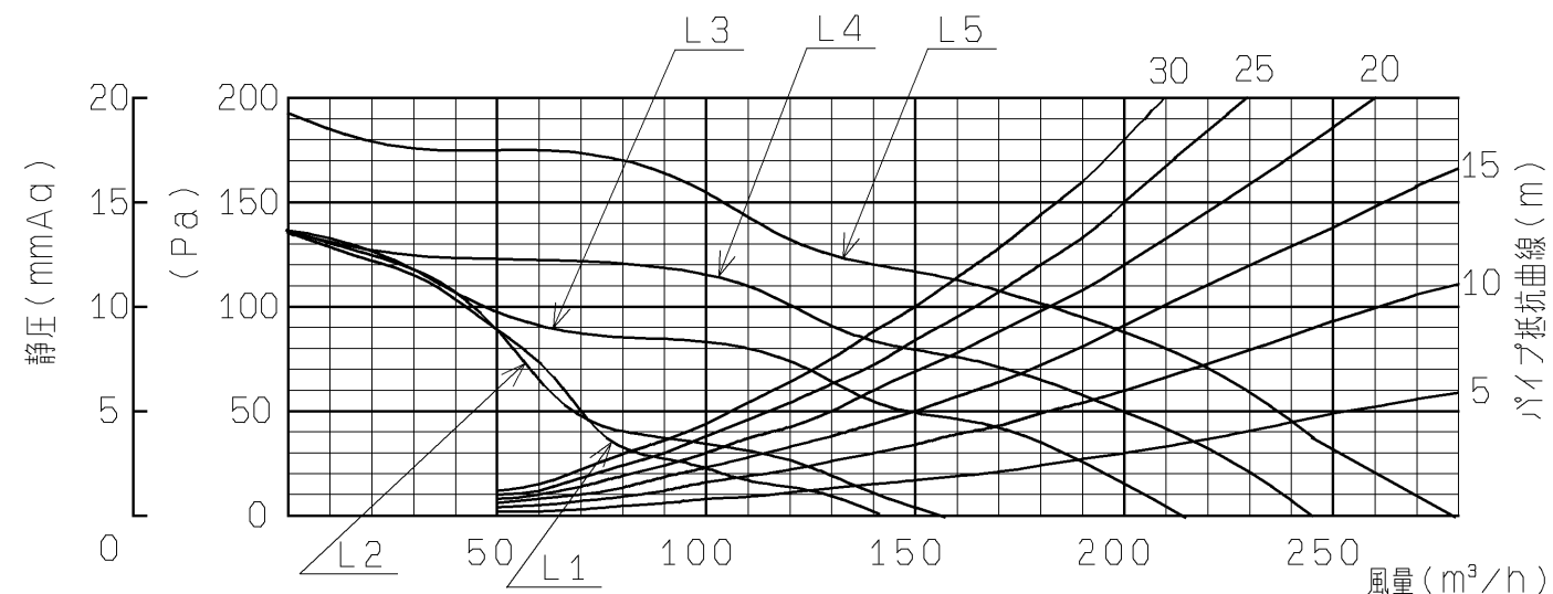
静圧風量特性曲線（24時間換気+トイレ換気運転時）
