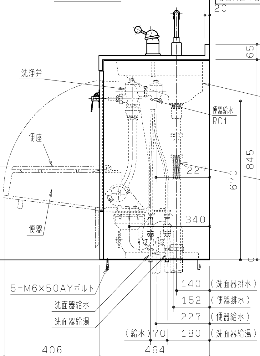
本体架台床固定位置
