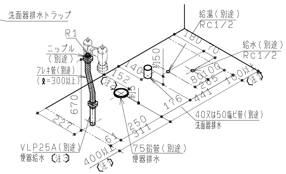
配管ナ上げ竹置図（別途手配，別途工事ください）
