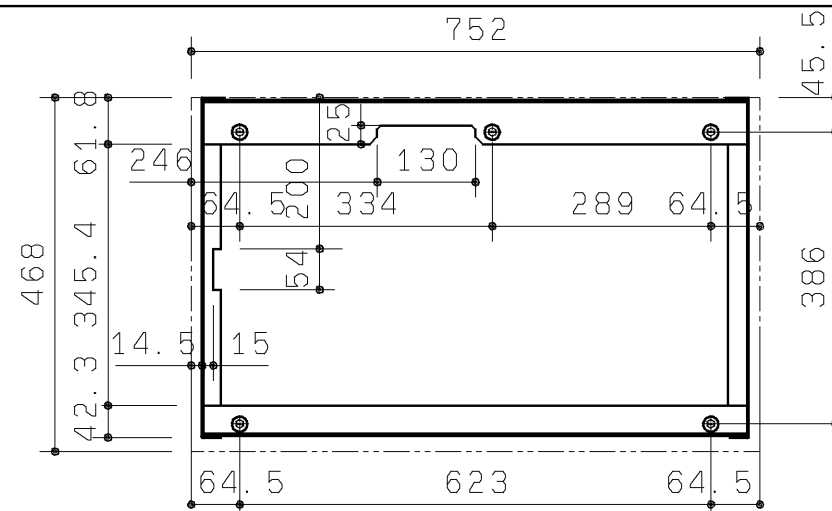
本体架台床固定位置
