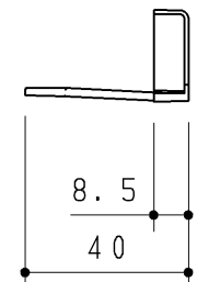
カウンターキャップセット
