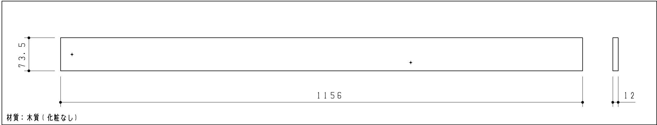
下段補強棒
