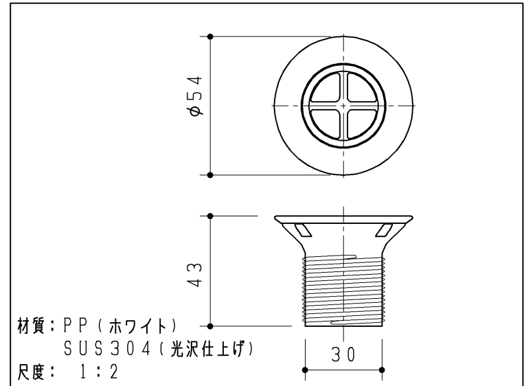
排水金具
