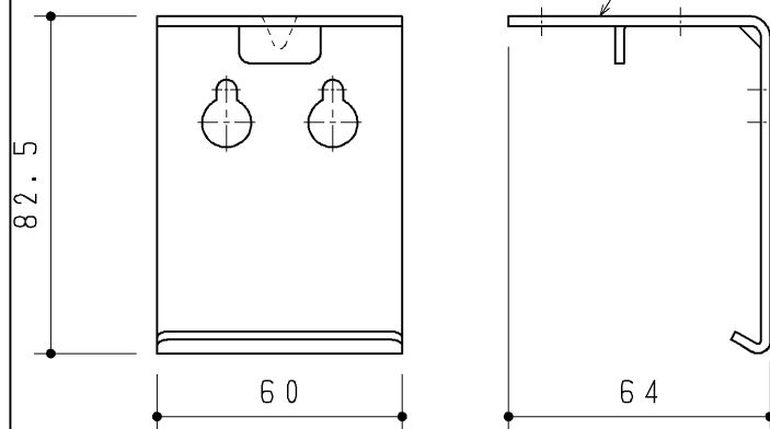
下段ブラケットセット
