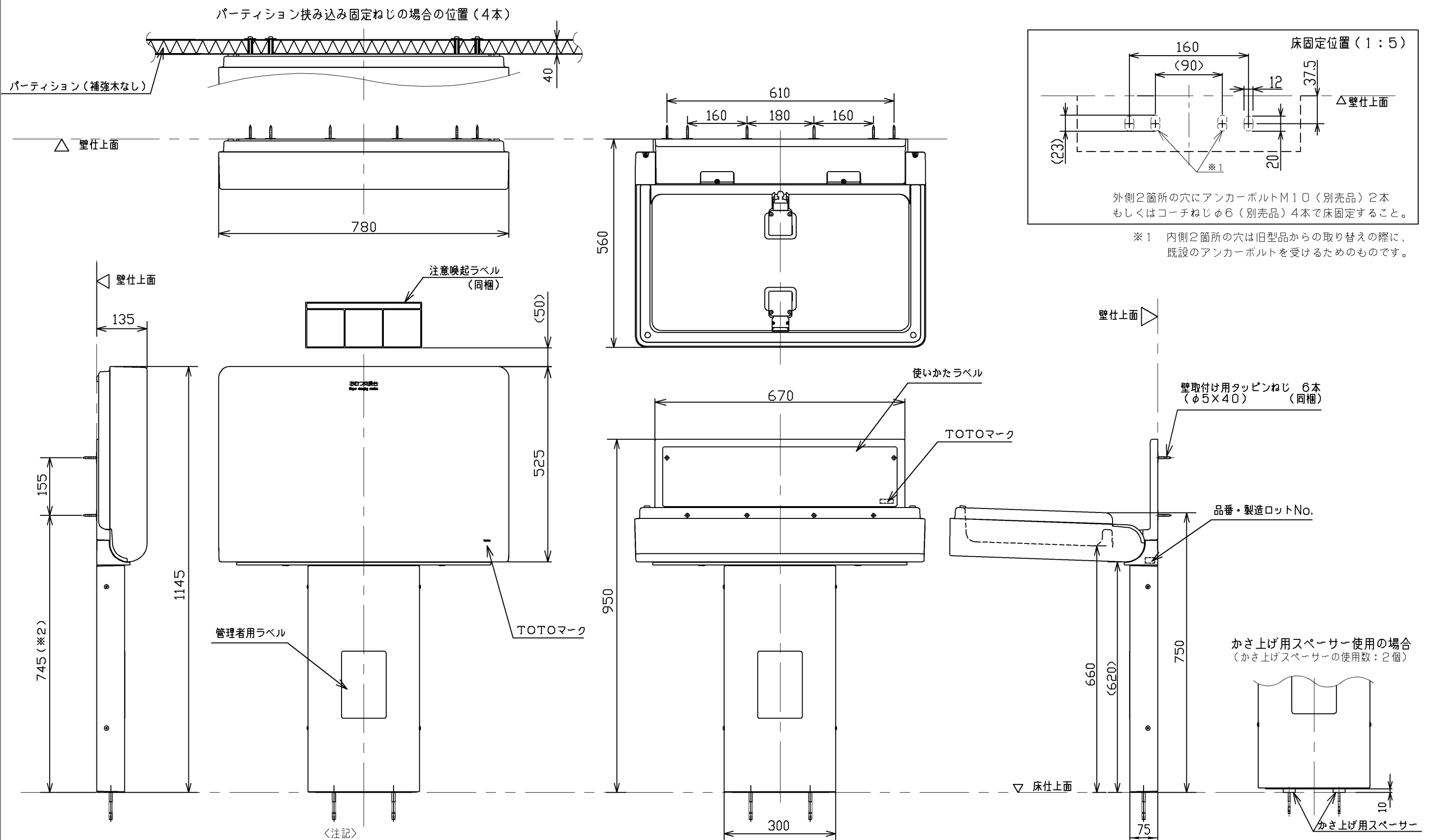
取付金具 (別売品) 各補強については2枚目参照のこと
