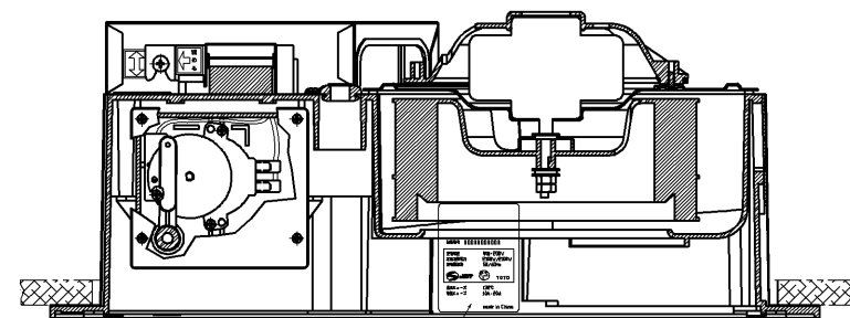
B-B断面
