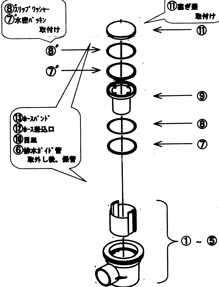
<塞ぎ蓋品B> 仕様図
