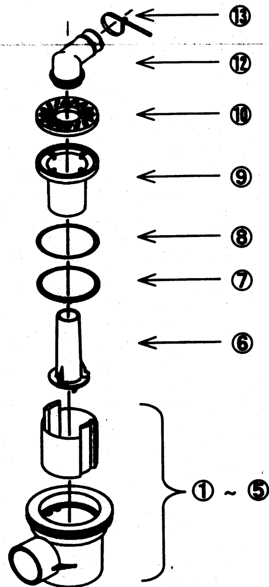
<正規品A> 仕様図
