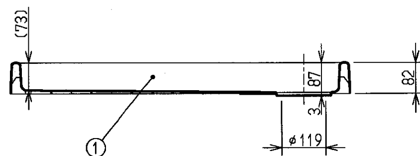
断面A-A
