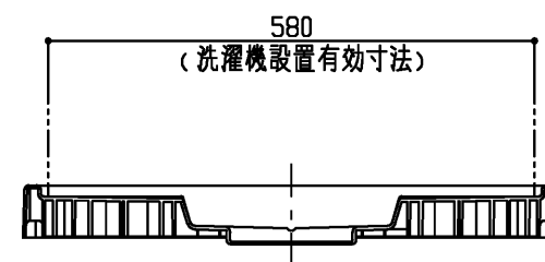
断面B-B
