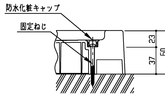
固定部詳細(尺度フリー)
