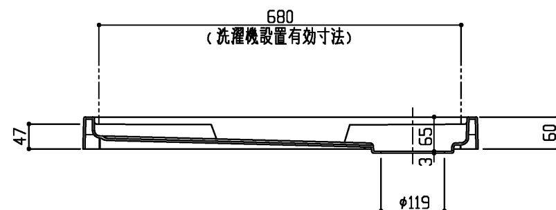
断面A-A
