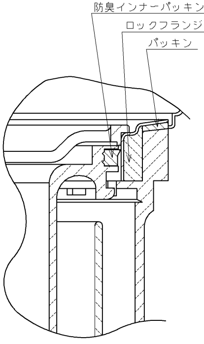
C部詳細図 (1:1)
