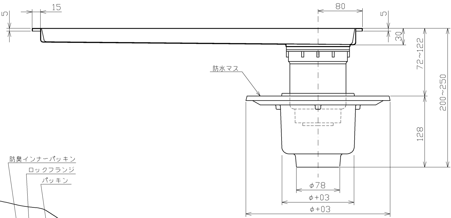
A-A' 断面 (排水ユニット本体)
