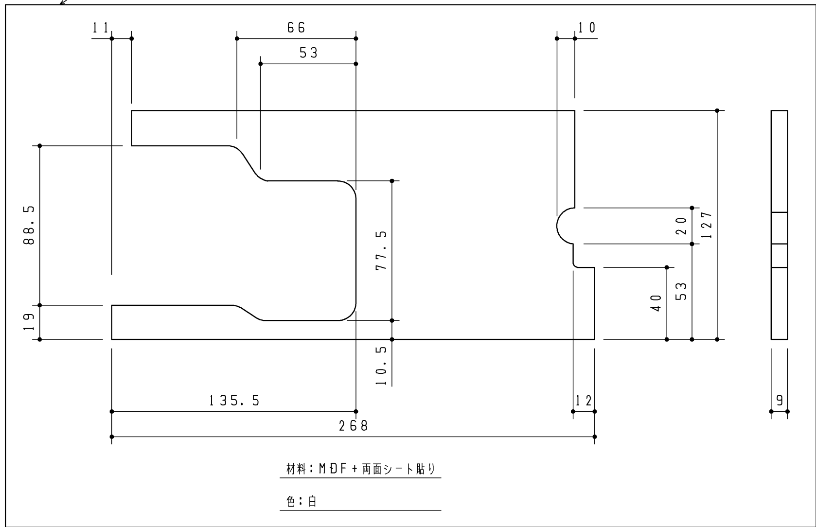
底板 (1ヶ)
