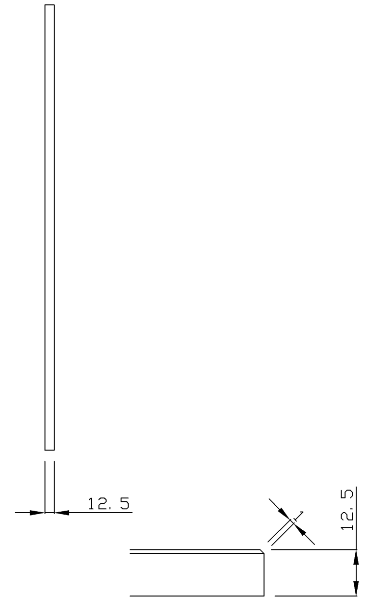
A部（面取り部）拡大図
