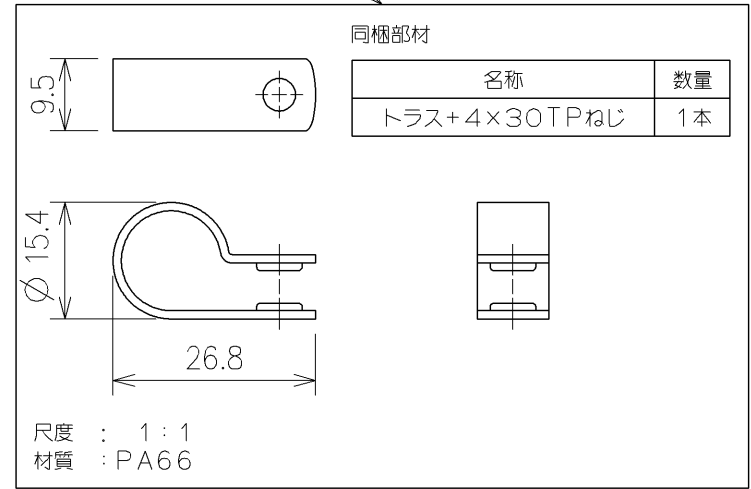
ホースクランプセット
