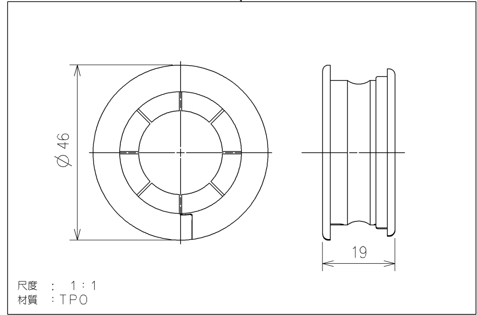
ホースクランプセット
