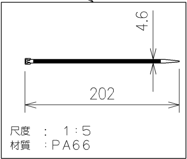
結束バンド(2ヶ)
