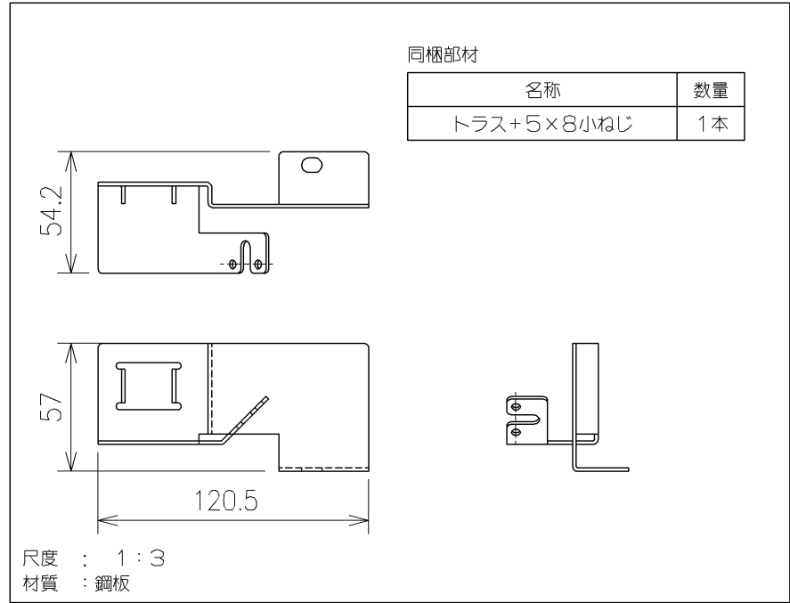
キャップセット
