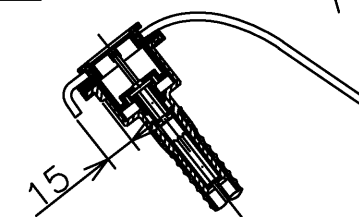
断面A-A(1:5)
