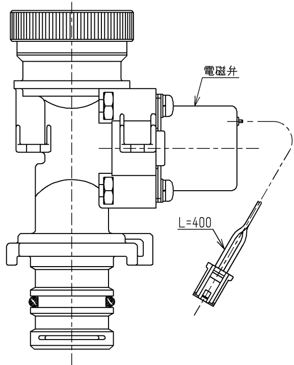
駆動部
