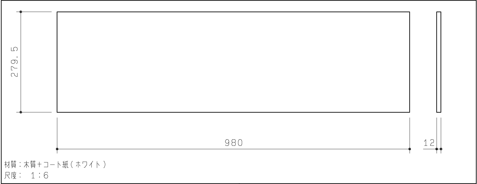
収納底板
