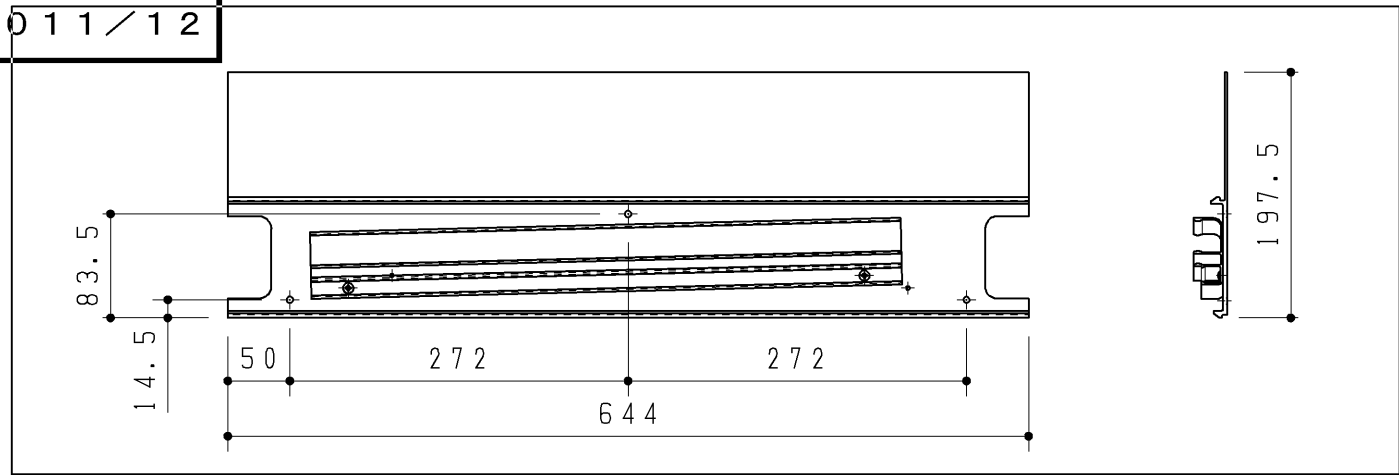
配管カバー
