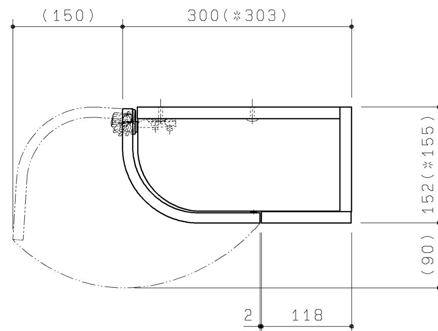
開口状態図
