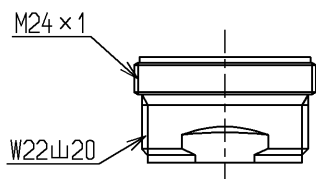
先端浄水器用(1:1)
