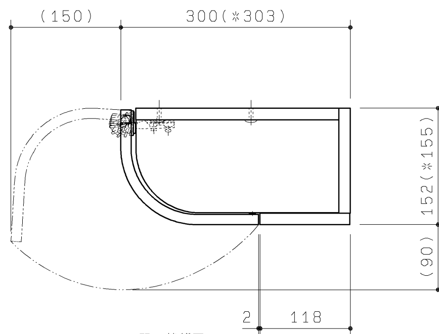
開口状態図
