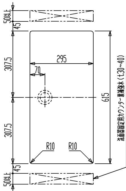
カウンター切込寸法
